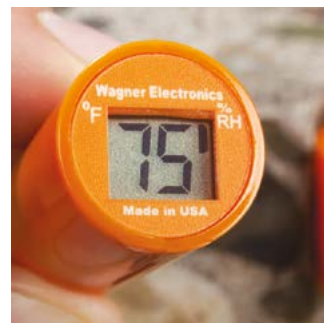
Der RH-Test (relative Betonluftfeuchte)
